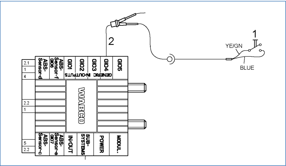
Utdrag ur schema 841 802 274 0
